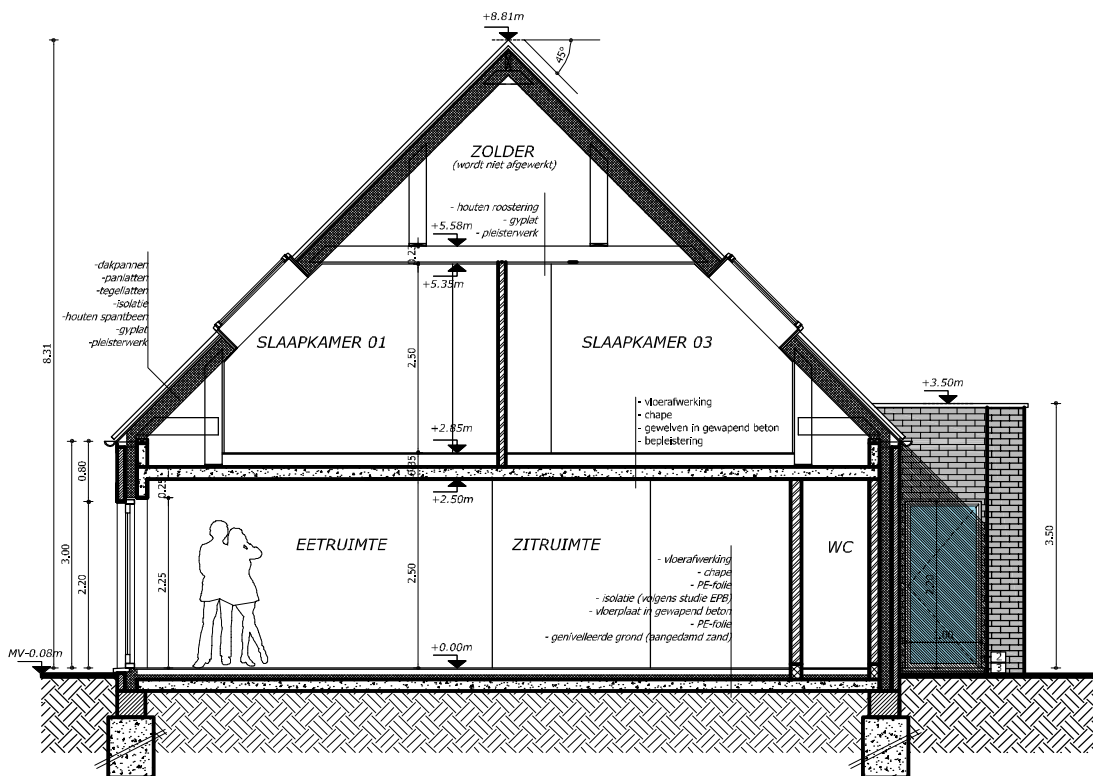
DOORSNEDIE AA'' SCHAAL 1:500
